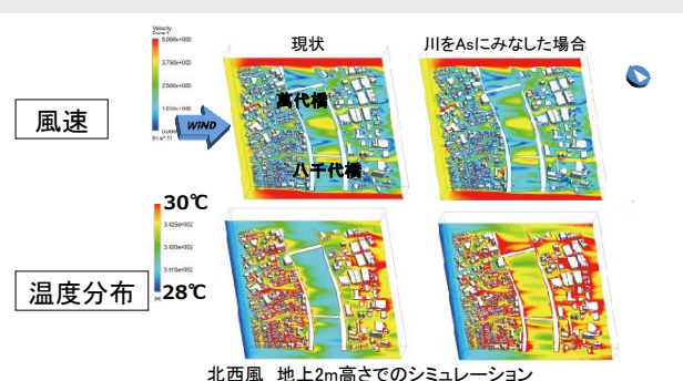
萬代橋周辺の温熱・風環境シミュレーション
